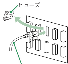
平型ヒューズタイプ電源取り出しコード
