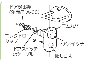
ドア部詳細
