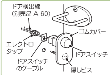
ドア部詳細
