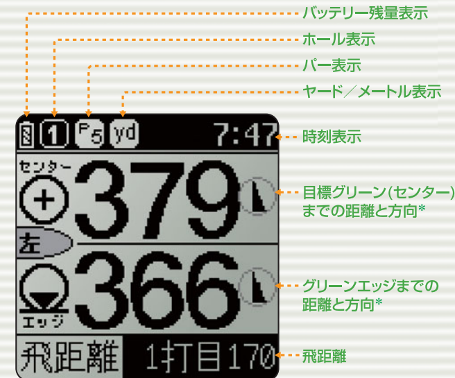
AGN1100のナビ画面(グリーンモード)
