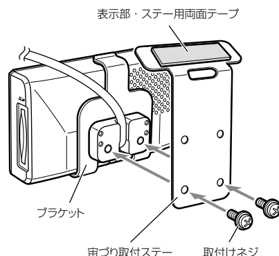
宙ぶり取付ステー
