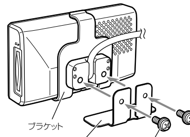
ダッシュボード 取付ステー
